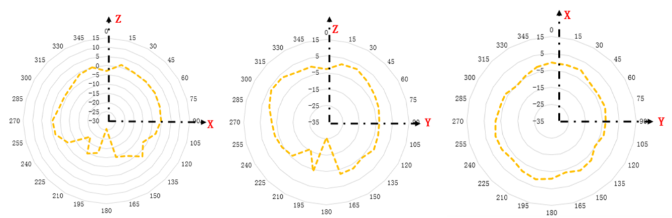
图 3. BLE 天线向量图
